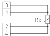
1x Vierleiterschaltung
