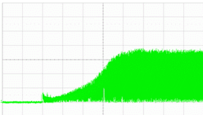
Anlaufstrom @ 24 V (I = 500mA/div ; t = 2s/div)
