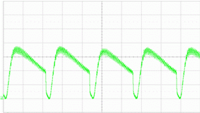
Laufstrom @ 24 V (I = 500mA/div ; t = 1ms/div)
