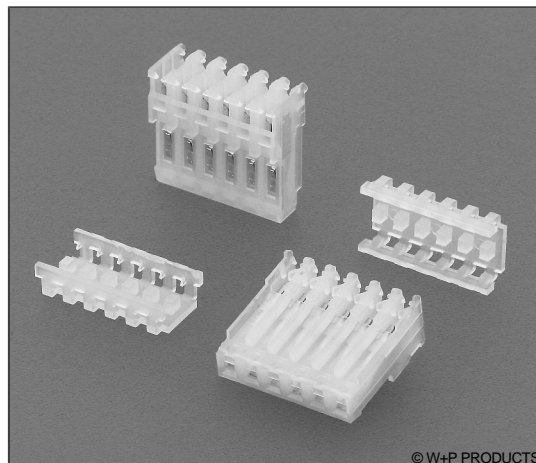
Cap
