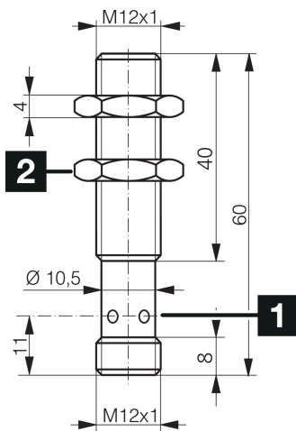
1) LED 4 x 90° (gelb) 2) Schlüsselweite 17 mm BK: schwarz BN: braun BU: blau
