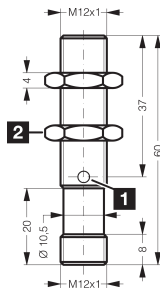
1) LED 2) Ouverture de clé 17 mm BK: noir BN: marron BU: bleu
