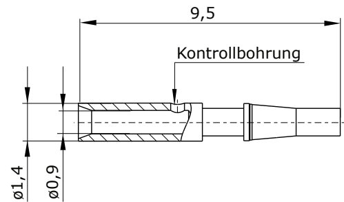
Hauptabmessungen Kontaktbuchse
